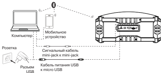
Рис. 4. Схема подключения
