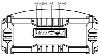
Рис. 3. Задняя панель
