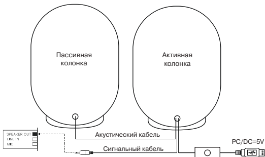
Рис. 2. Схема подключения
