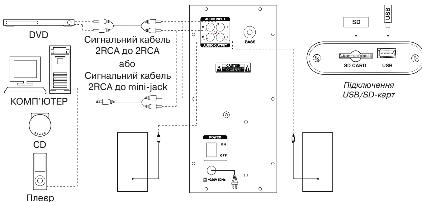
Мал. 5. Схема підключення
