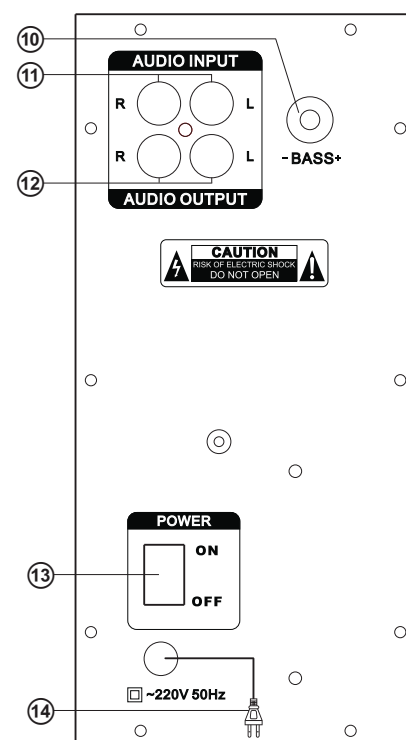
Мал. 2. Задня панель
