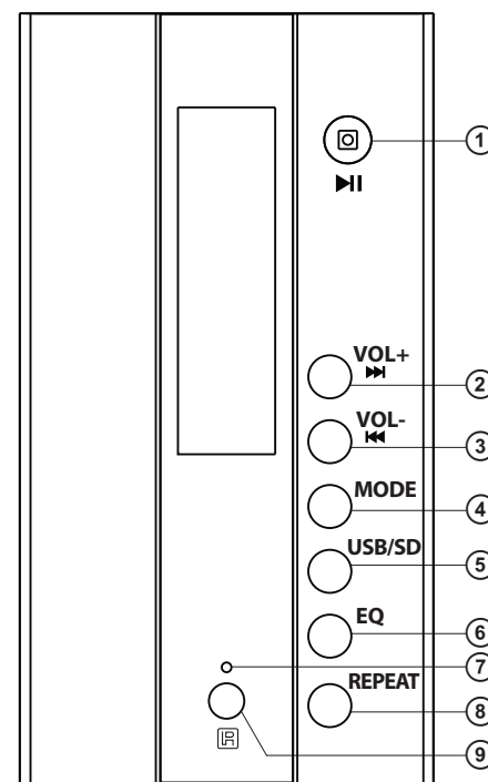
Рис. 1. Передняя панель
