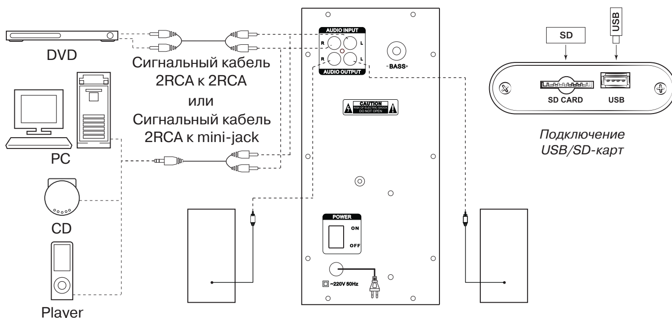
Рис. 5. Схема подключения
