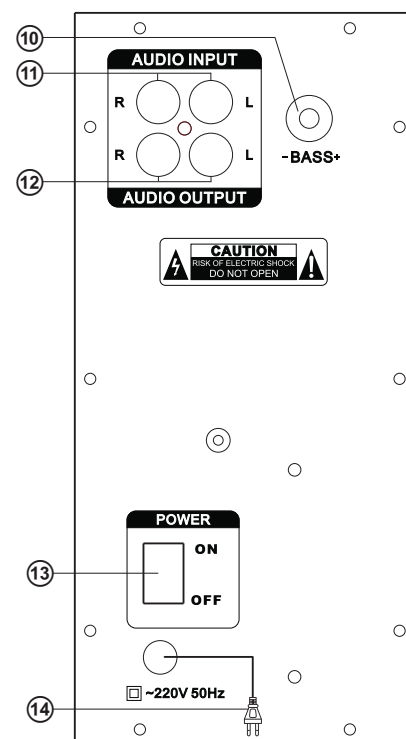
Рис. 2. Задняя панель
