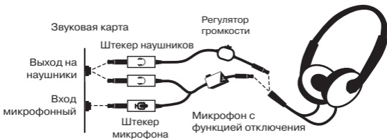
Рис. 1. Схема подключения
