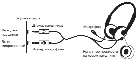
Рис. 1. Схема подключения
