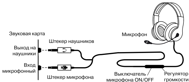
Рис. 1. Схема подключения
