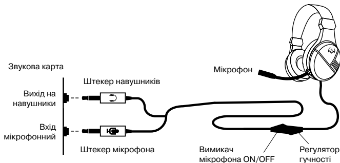
Мал. 1. Схема підключення
