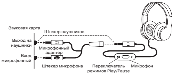
Рис. 1. Схема подключения
