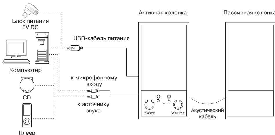
Рис. 2. Схема подключения
