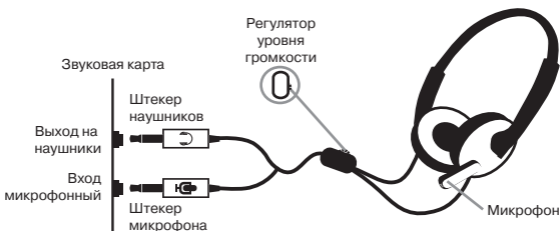
Рис. 1. Схема подключения
