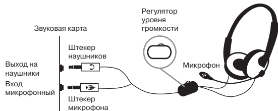
Рис. 1. Схема подключения
