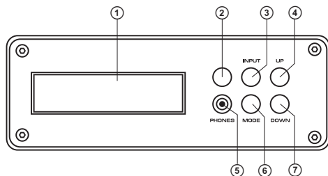
Рис. 2. Панель управления активной колонки
