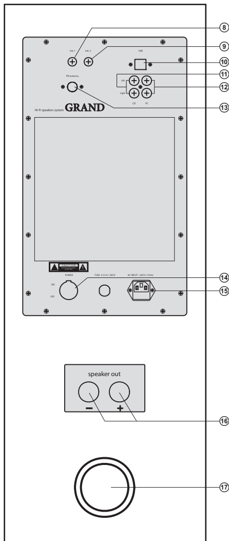
Рис. 3. Задняя панель активной колонки
