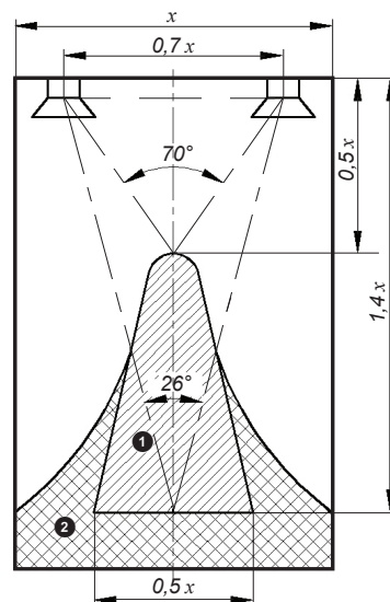
Рис. 1. Схема расположения АС
