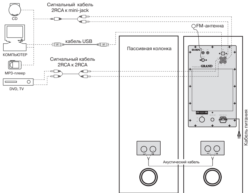
Рис. 5. Схема подключения
