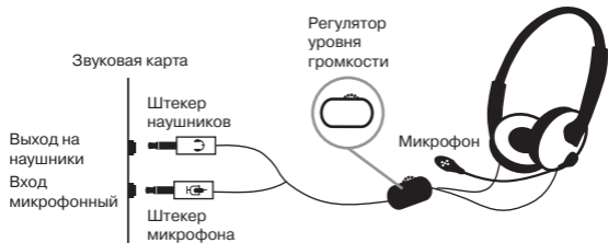
Рис. 1. Схема подключения
