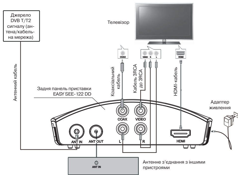
Мал. 5. Схема підключення
