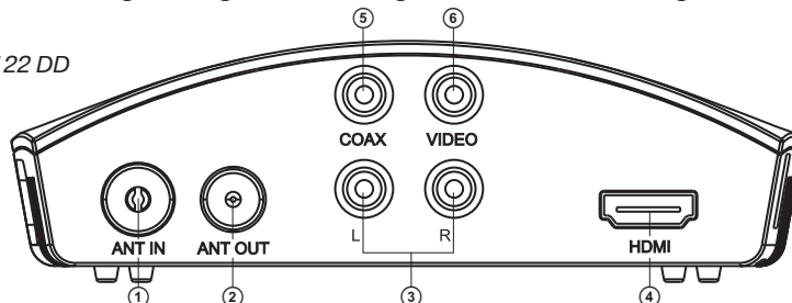
Мал. 3. Задні панелі EASY SEE-121 та EASY SEE-122 DD
