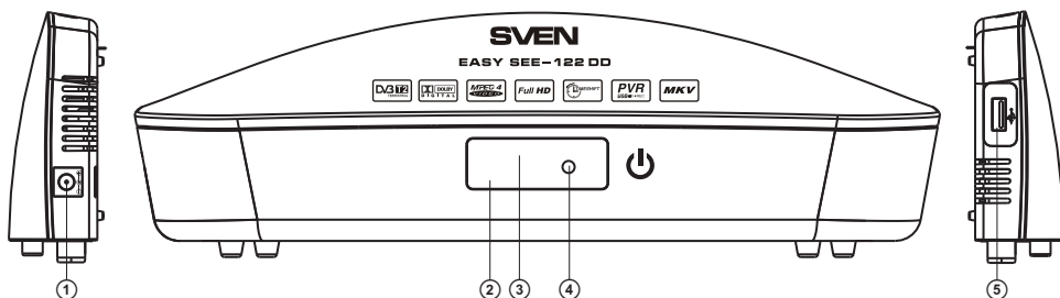
Мал. 2. Бічні та передня панелі EASY SEE-122 DD
