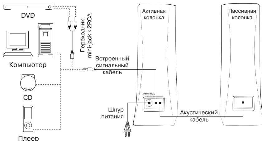
Рис. 2. Схема подключения
