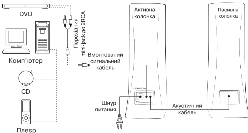
Мал. 2. Схема підключення
