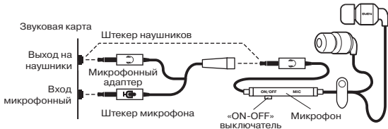
Рис. 1. Схема подключения
