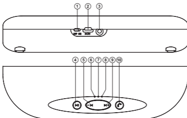
Рис. 1. Конструкция AC
