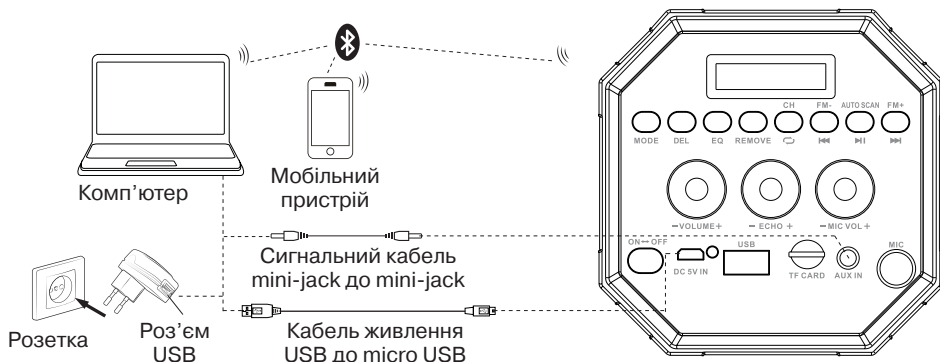
Мал. 2. Схема підключення
