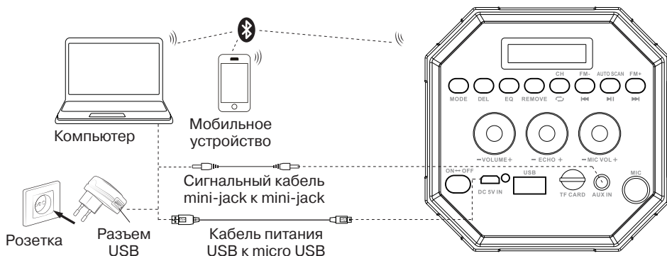
Рис. 2. Схема подключения
