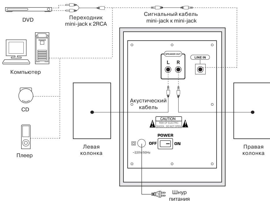
Рис. 3. Схема подключения
