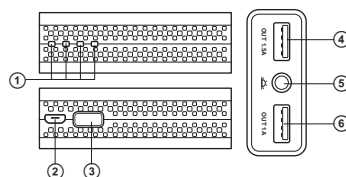
Рис. 1. Устройство батареи
