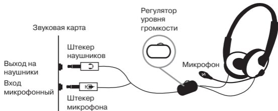
Рис. 1. Схема подключения
