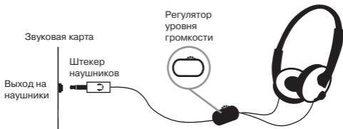
Рис. 1. Схема подключения
