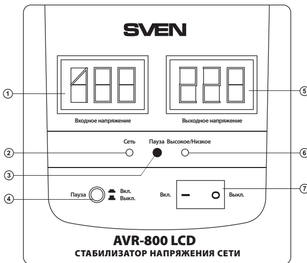
Рис. 1. Передняя панель
