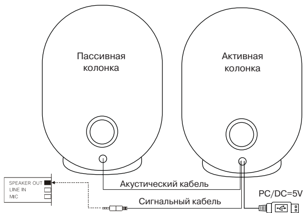
Рис. 2. Схема подключения
